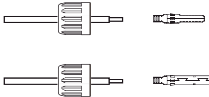
Abbildung 4.9 Einführen des Kabels in die Überwurfmutter des Steckers und den Kontaktstift
