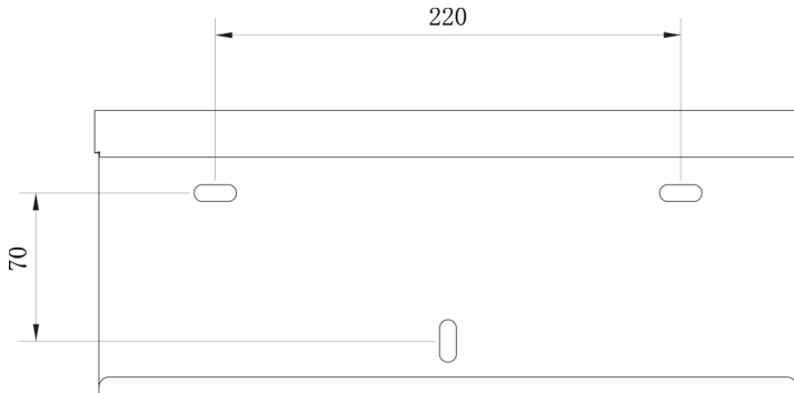
Abbildung 4.3 Wandmontage des Wechselrichters
