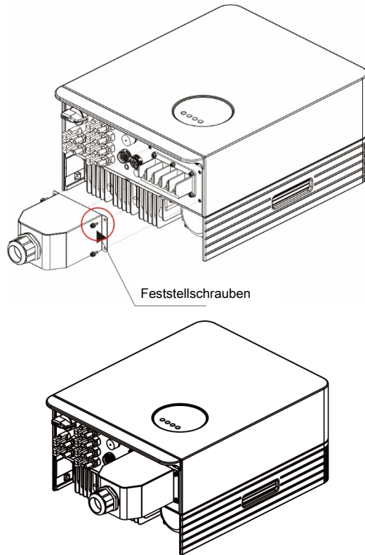
Abbildung 4.13 Anschluss des AC-Steckers an den Wechselrichter
