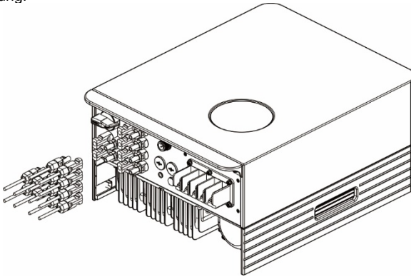
Abbildung 4.12 Anschluss der DC-Steckverbinder an den Wechselrichter
